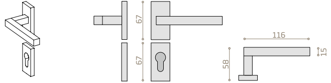
L porte plaque carrée
