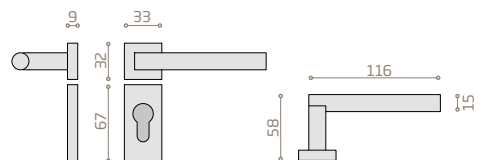
L porte plaque carrée
