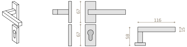
L Türeckige Rosette
