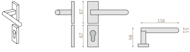
L Türeckige Rosette
