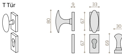
T Türeckige Rosette
