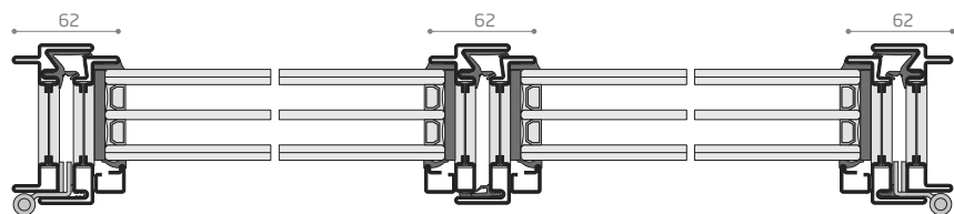
Porta a due ante con nodi costanti su tutto il perimetro, compreso nodo centrale e sezione a pavimento.
