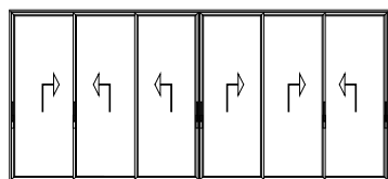
Schema | Type E3 - F3
