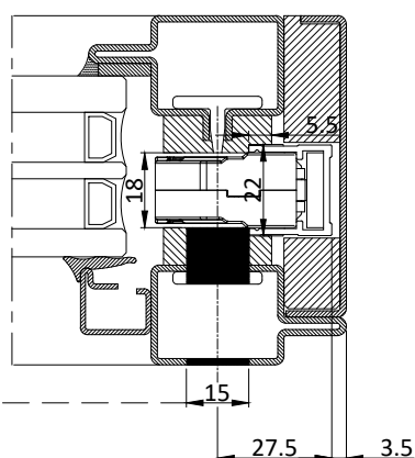
sezione | section A cremonese cremone
